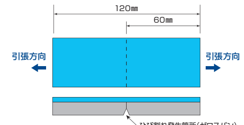
JHS 417-1999 日本道路公園規格「コンクリート塗材の品質規格試験方法 4.7 ひび割れ追従性試験」準拠
